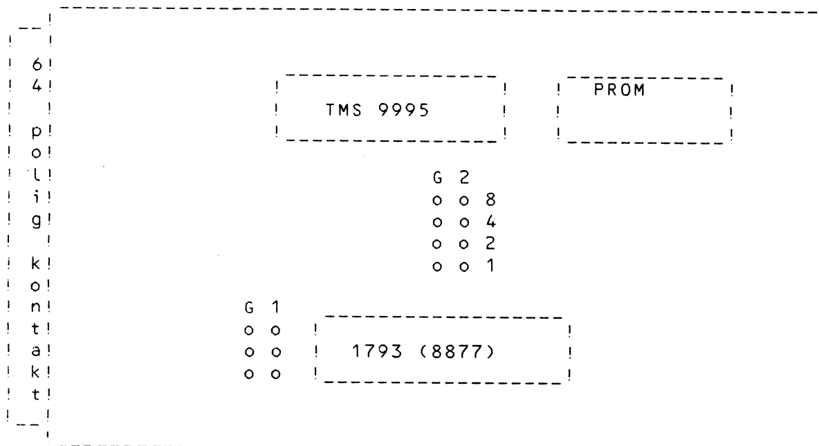
Figur 1: Placering av bygelgrupperna G1 och G2
